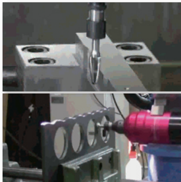
※画像提供 カトウ工機(株)DBR7-P 型バリ取りホルダー
